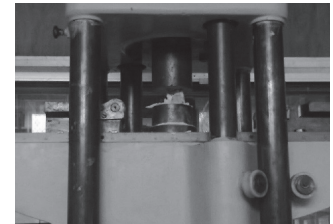
Figura 11. Ensayo de compresión uniaxial al travertino tipo Puebla. Página 17.
